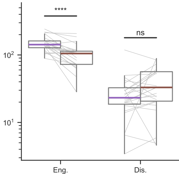
2AFC
