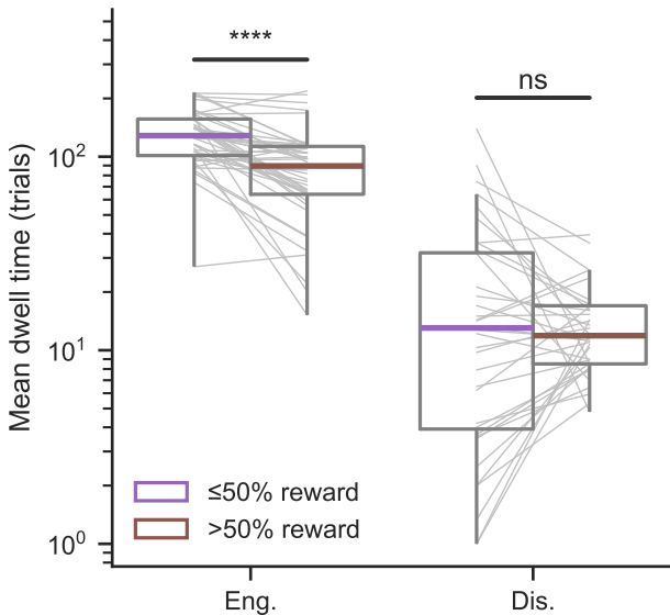
2ADC
